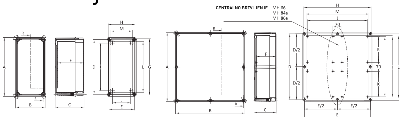
Dimenzije kutija (mm)
