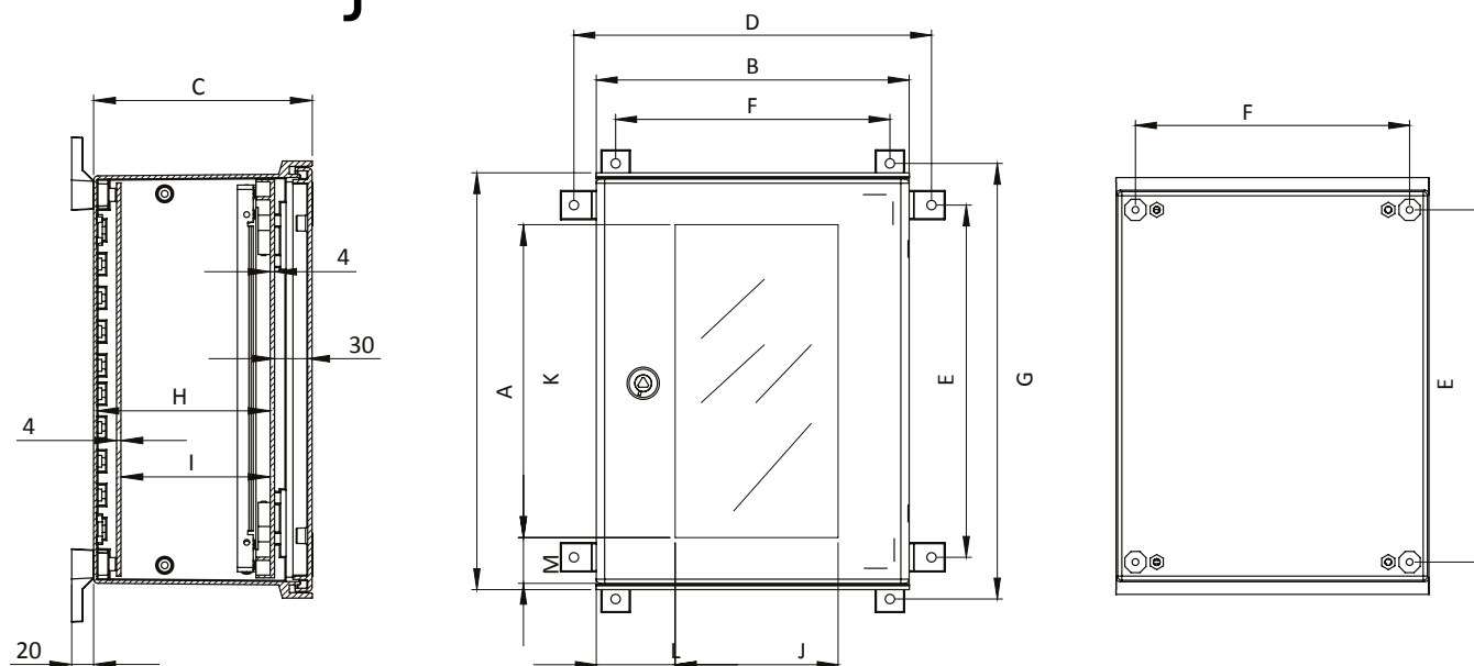
Dimenzije ormara (mm)
