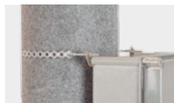
Montaža na stup Ref. 06CAFP0100
